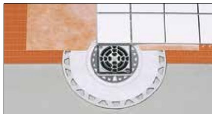
Schlüter®-KERDI-DRAIN systém podlahových vpustí pro bezpečné napojení kontaktních izolací Schlüter®-KERDI nebo ostatních kontaktních izolačních systémů na odvodnění
