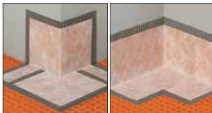
Schlüter®-KERDI-KERECK předpřipravené vnější rohy
