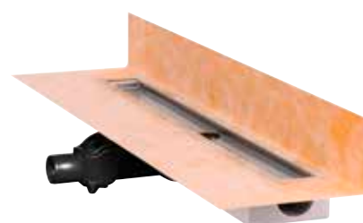
Schlüter-KERDI manžeta, postavená pro montáž ke stěně
