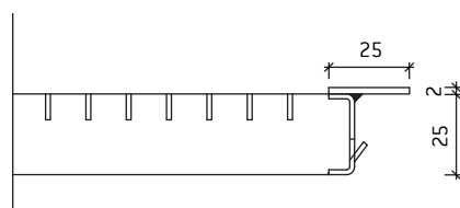
Světelný rošt s oky 30/10 Přejezdový osobními vozidly, s ochranou hranou
