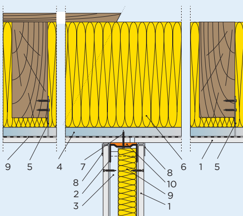
Detail napojení příček v podkroví
