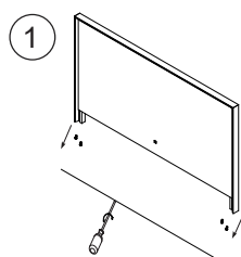
1. Vjměte šrouby z rámu.
