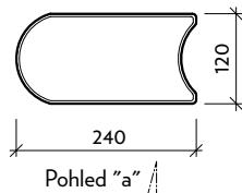
Půdorys
