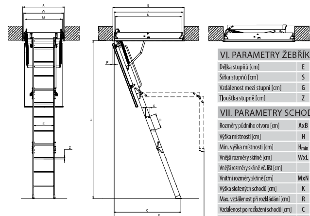
V. SCHÉMA SCHODŮ LWZ Plus
