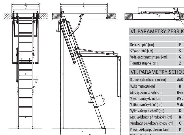
V. SCHÉMA SCHODŮ LWL Extra
