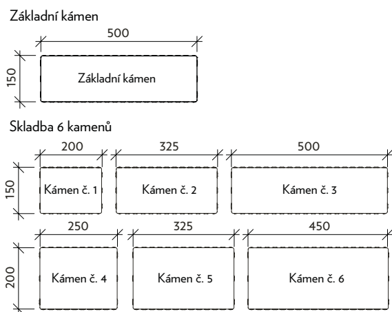
Půdorys
