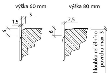
Řez hranou - hladký povrch
