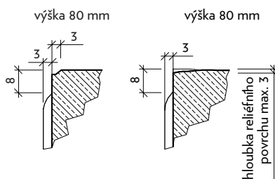
Řez hranou - reliéfní povrch
