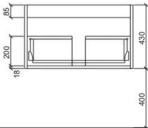
Pūdorys
