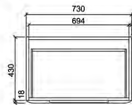
Púdorys
