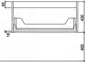
Pūdorys
