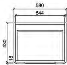
Pūdorys
