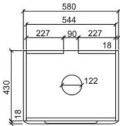
Púdorys
